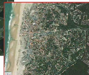
Secteur regroupant les enjeux concernés par le risque d'érosion nécessitant une relocalisation © BD Pigma
